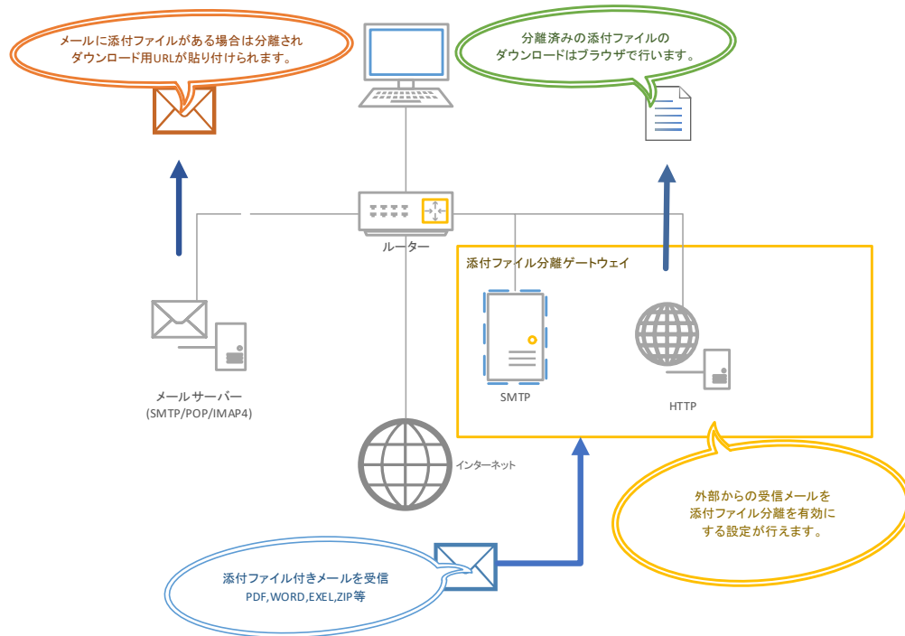
添付ファイル分離配送&ファイル受信通知機能 SMTPゲートウェイ構成図 外部から受信
